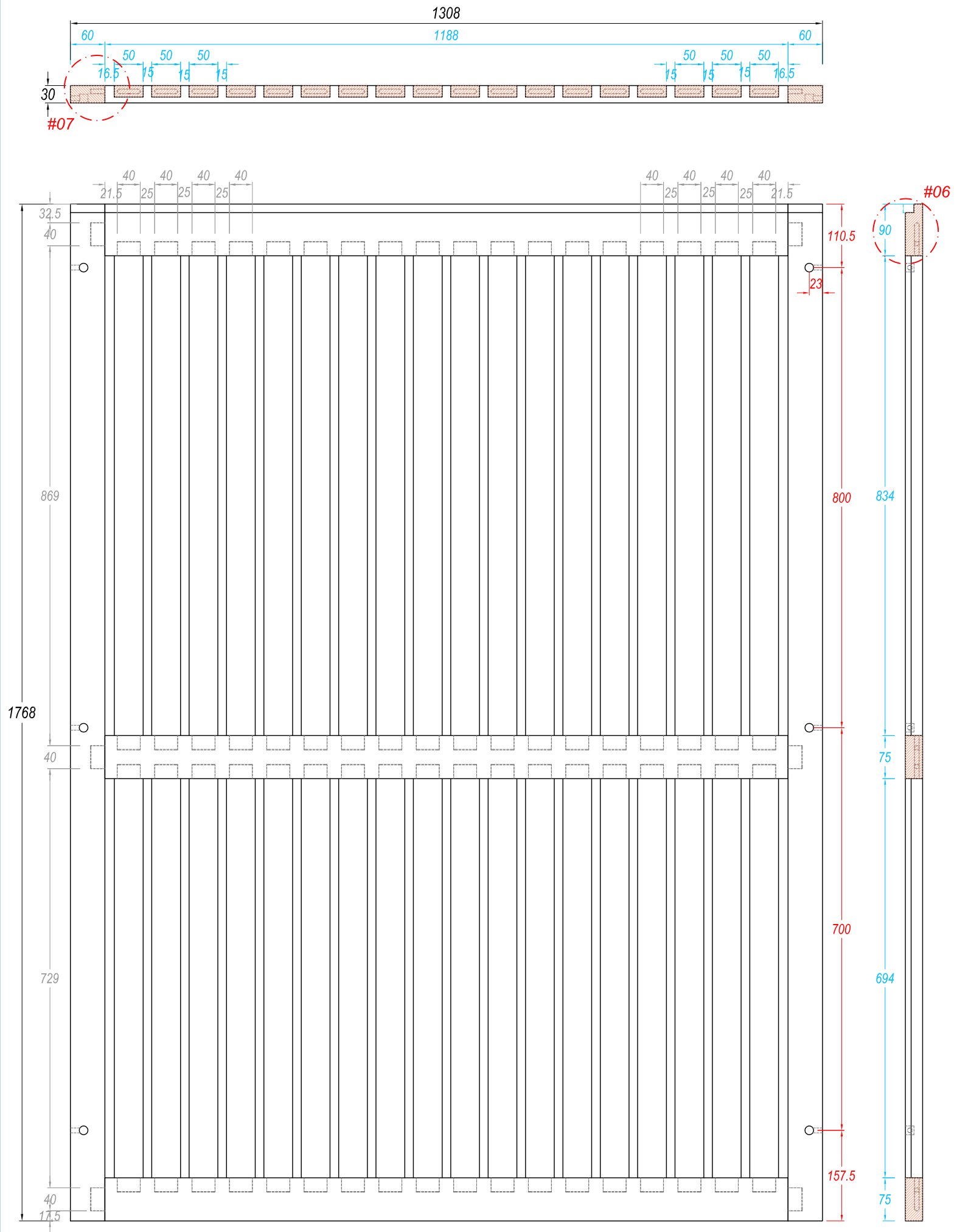
BACK FRAME Scale 1 : 8
