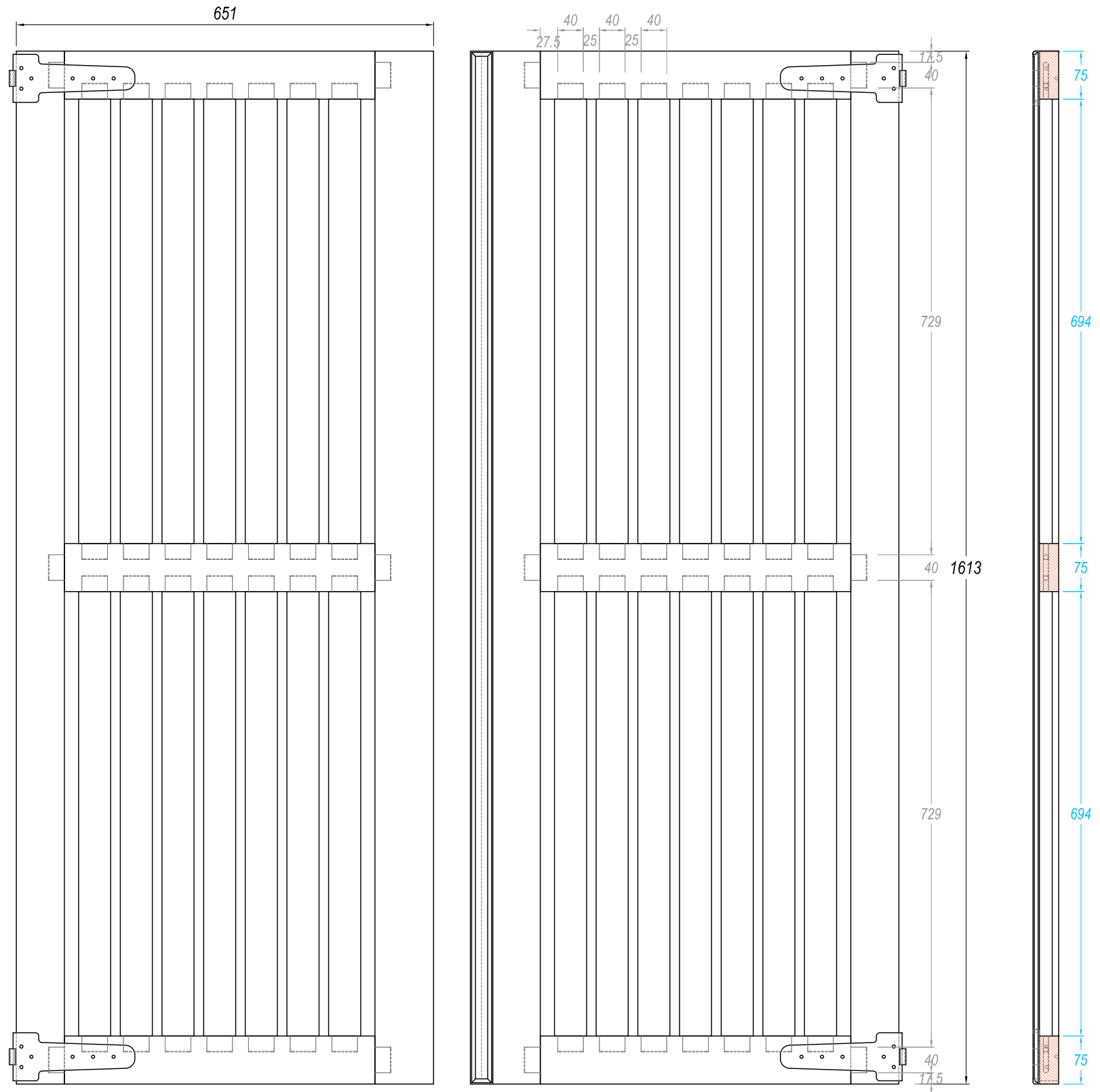
DOOR FRAME Scale 1 : 8
