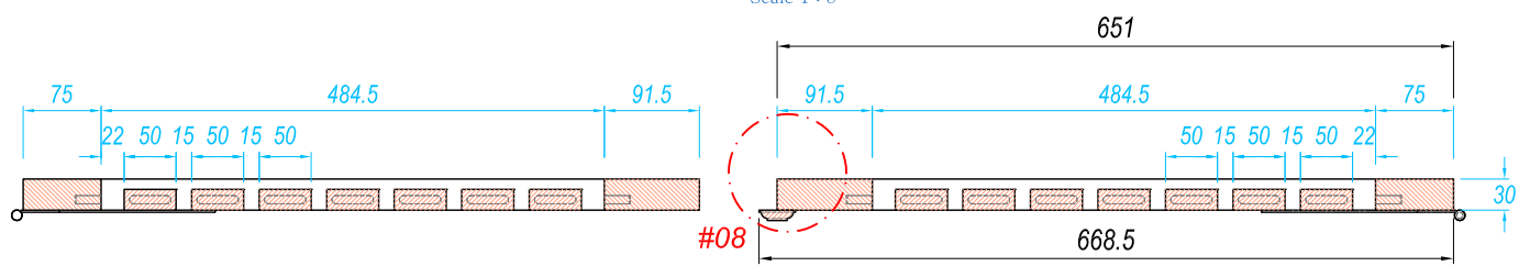
DOOR FRAME Scale 1 : 8
