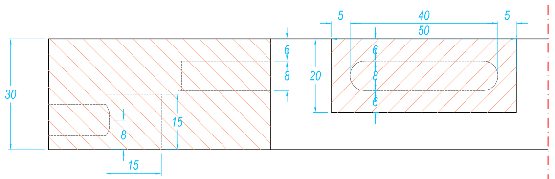
DETAIL #07 Scale 1 : 1
