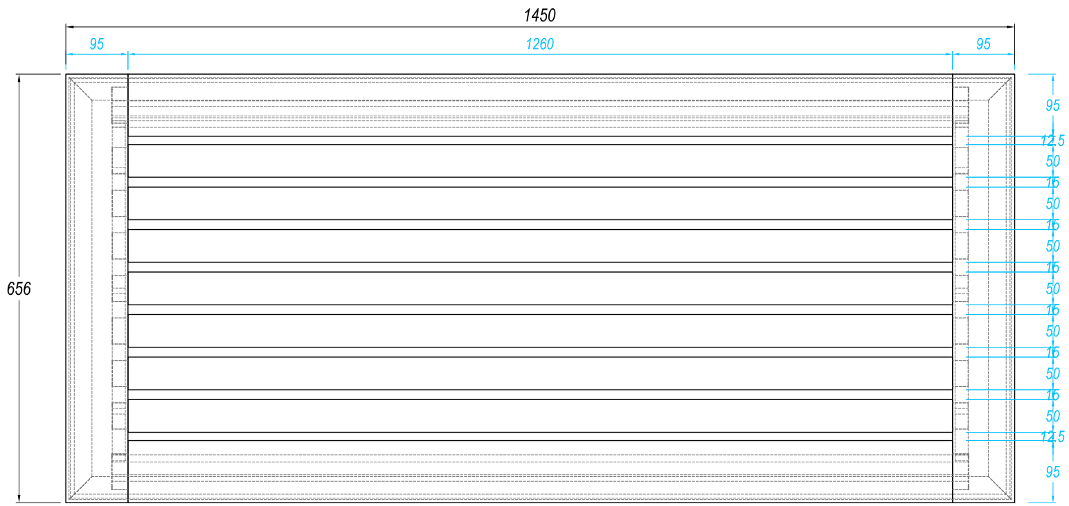
TOP FRAME Scale 1 : 8
